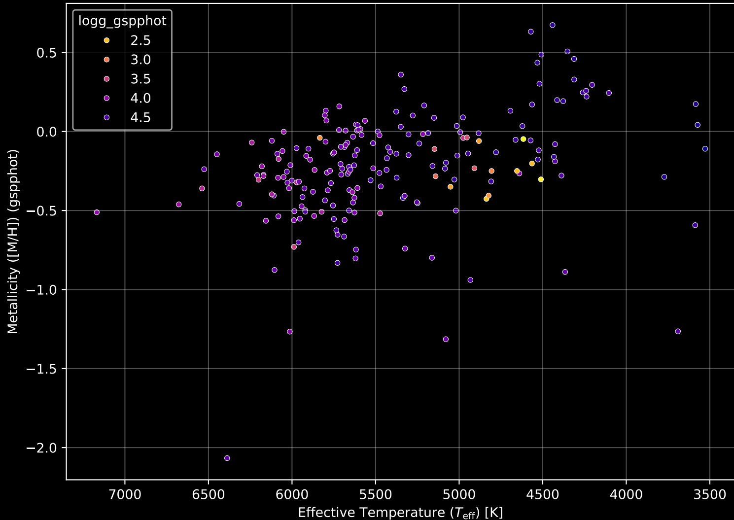
APOGEE DR17 Field: [180-75] Stellar Population Parameters (n= 199)
